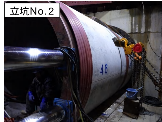
推進工法(ヒューム管布設)状況
