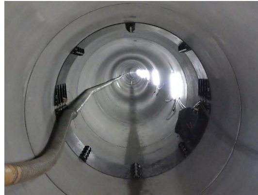
推進工法(U-M管布設完了)状況
