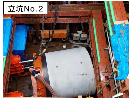
推進工法(U-M管布設)状況
