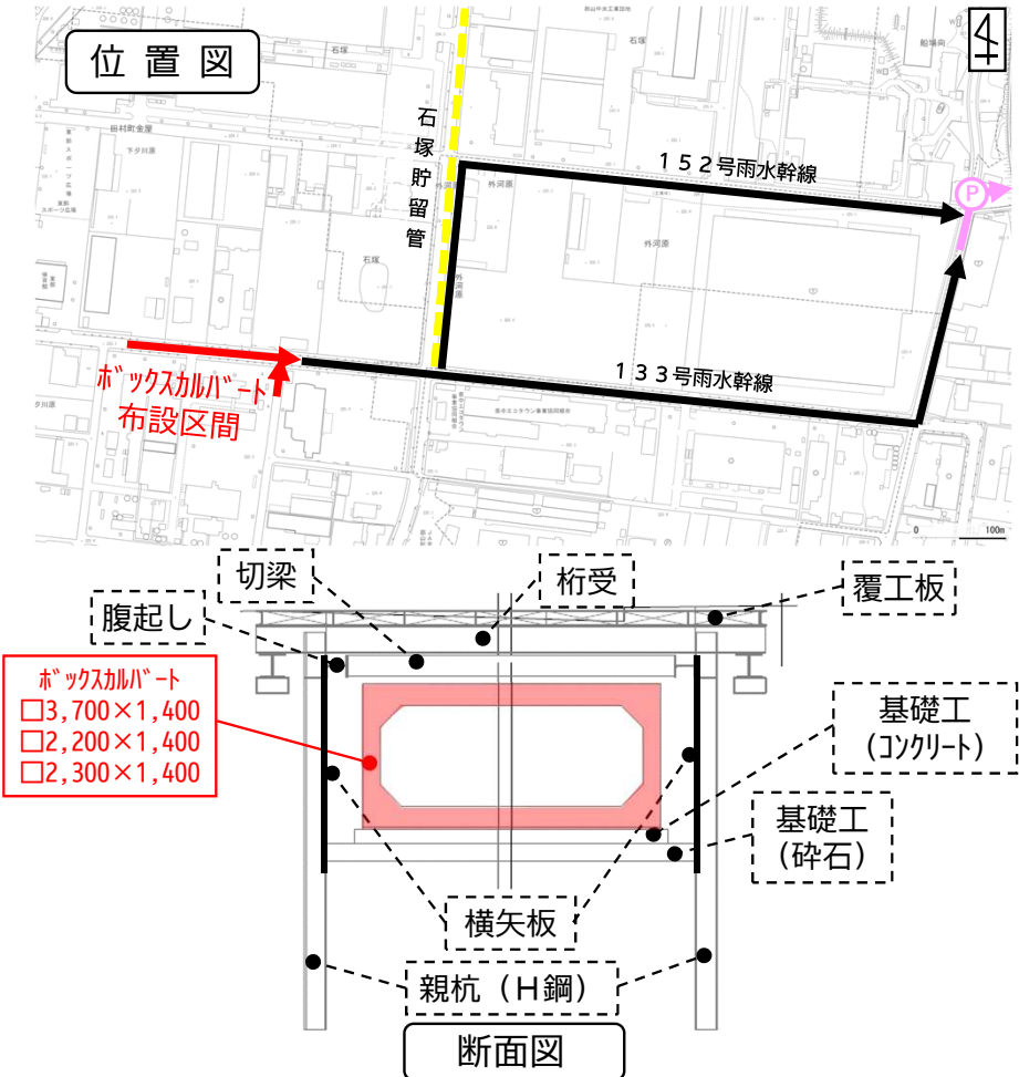
ボックスカルバート布設状況
