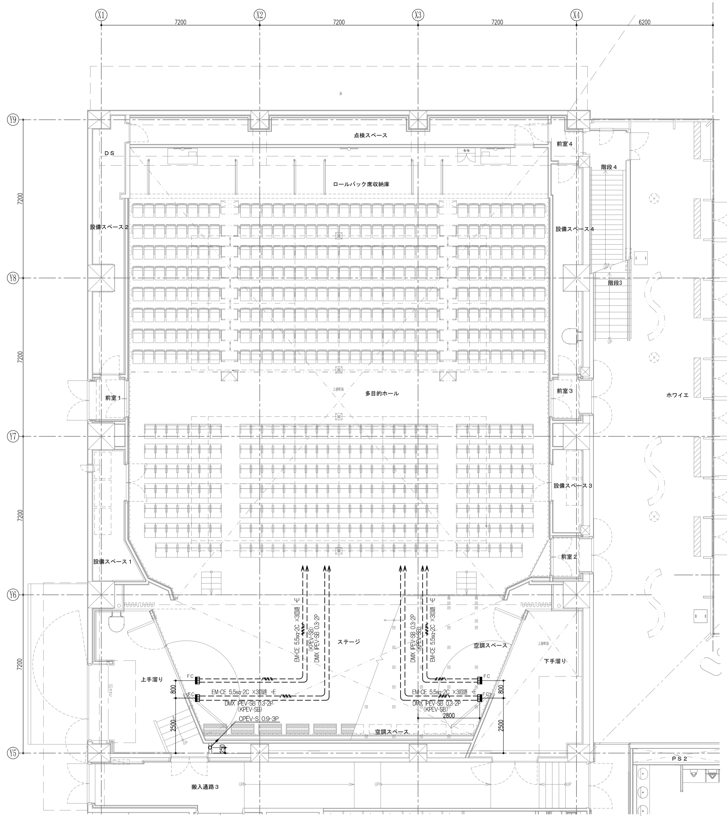
1階 平面図
