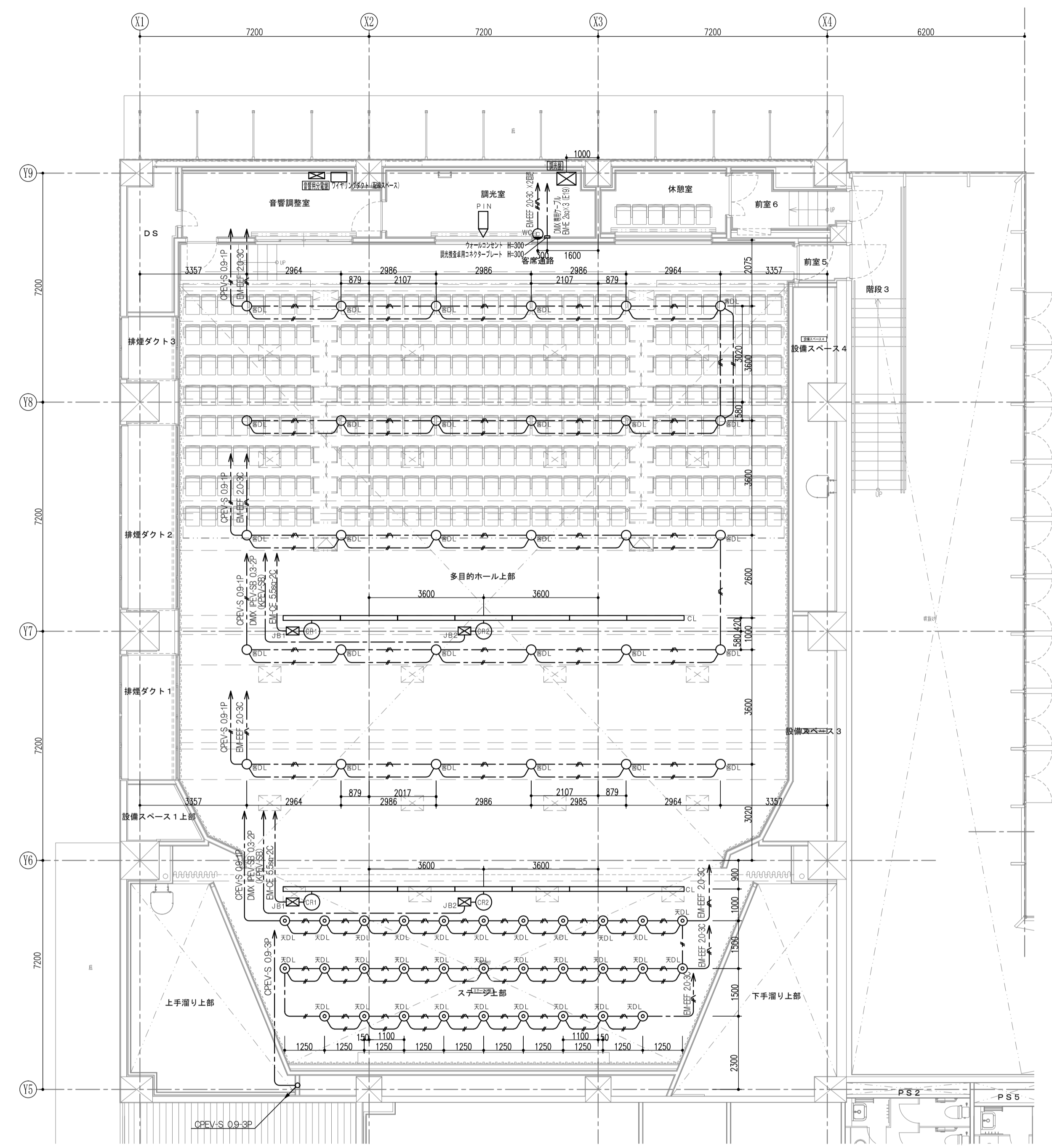
2階 平面図
