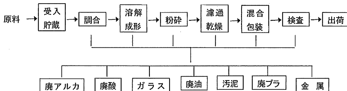
図1 フリット製造フローシート (No.1)
