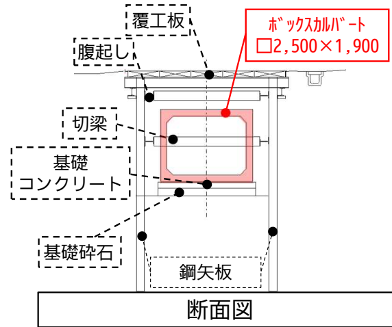
ボックスカルバート布設状況
