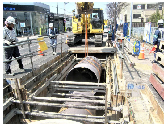
新設管布設状況
