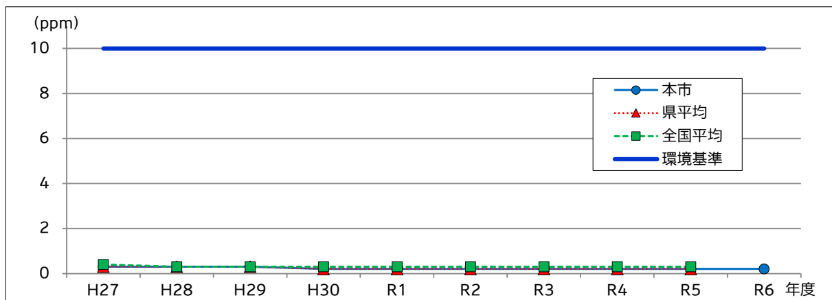
図 9 一酸化炭素濃度 (年平均値の推移)
