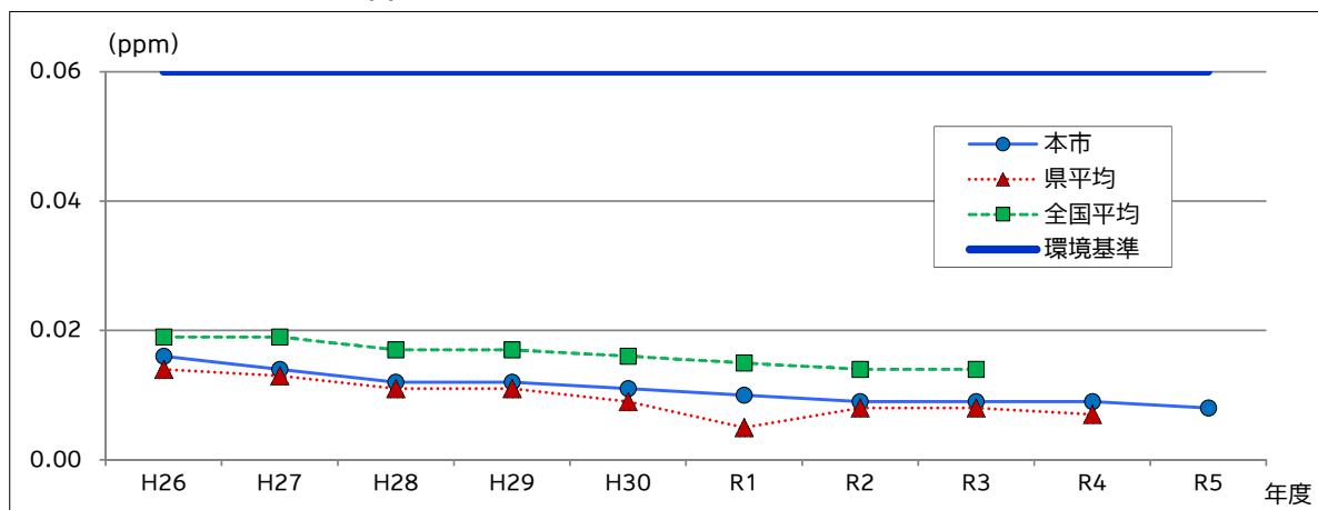
図7 二酸化窒素濃度（年平均値）の推移
