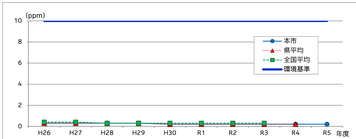
図 9 一酸化炭素濃度 (年平均値の推移)
