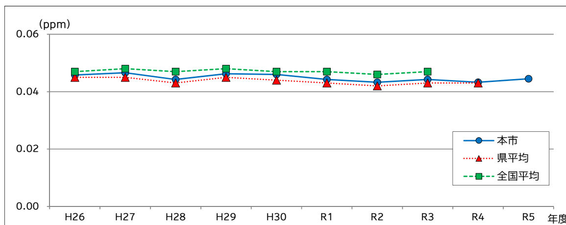
図3 光化学オキシダント濃度 (昼間の日最高1時間値の年平均値) の推移
