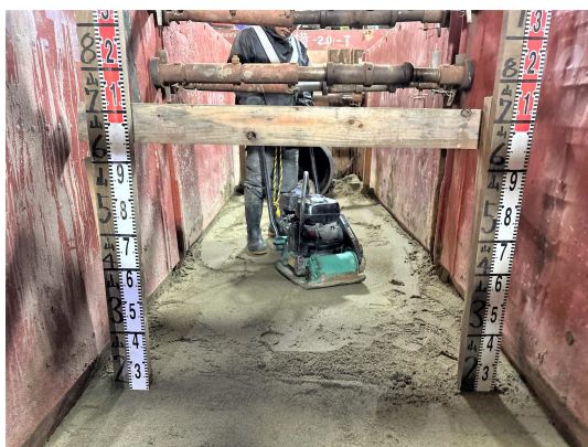
基礎砂転圧状況
