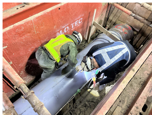
新設管布設状況
