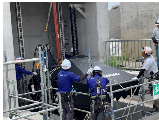
主ポンプ取付状況
