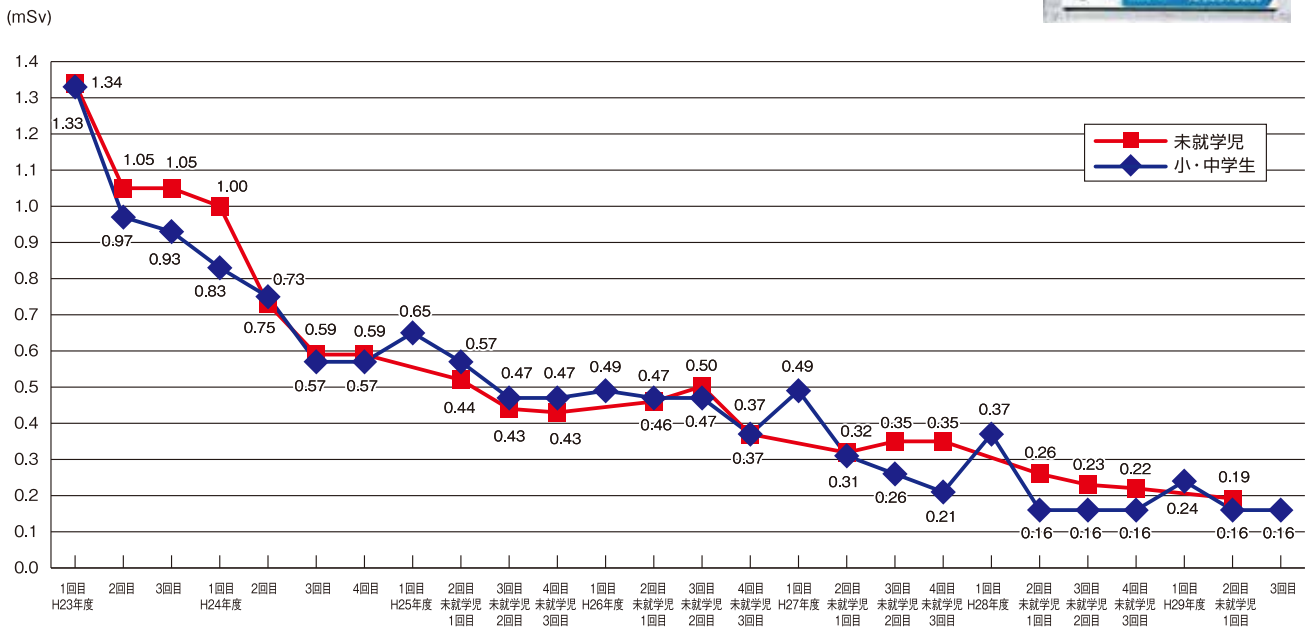
バッジ式積算線量計の測定結果の推移 (平均値を1年間に換算)
