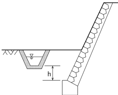
図 2(6)-3 水路に近接する場合の根入れ
