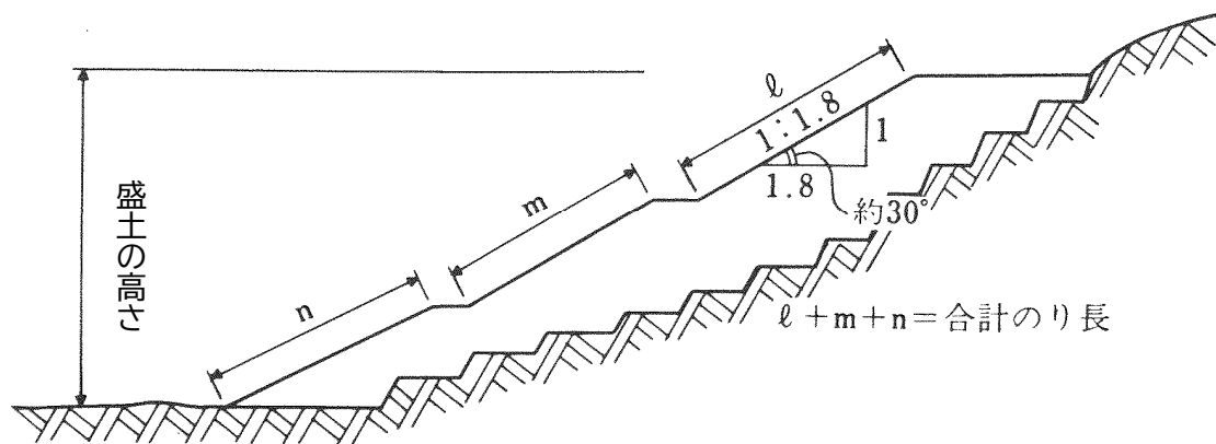
図 1(10)-1 盛土の高さ
