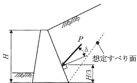
(a)重力式擁壁の場合
