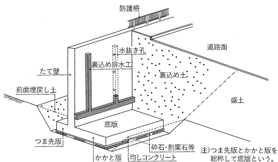
図 2(2)-1 擁壁各部の名称
