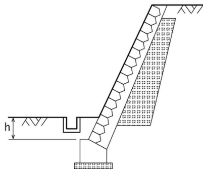
図 2(6)-4 U字溝に接する場合の根入れ
