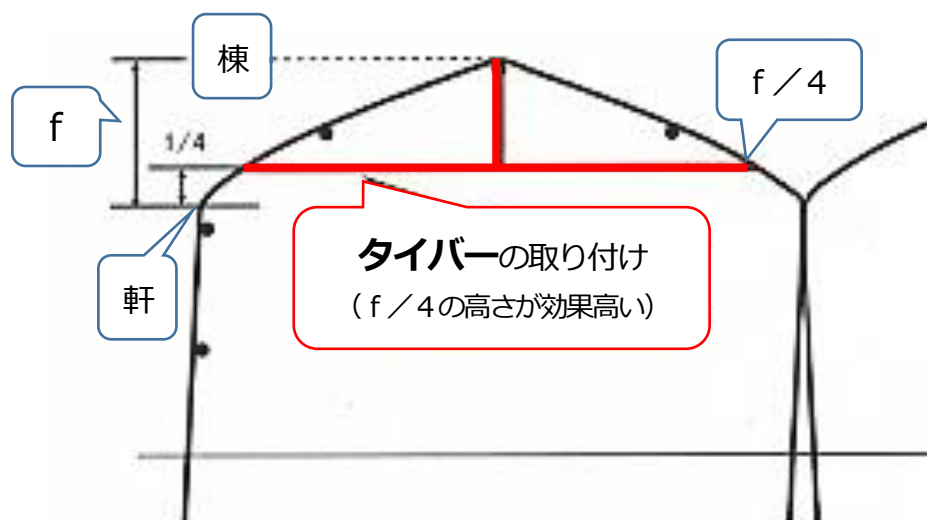
タイバーによる肩部の補強事例
