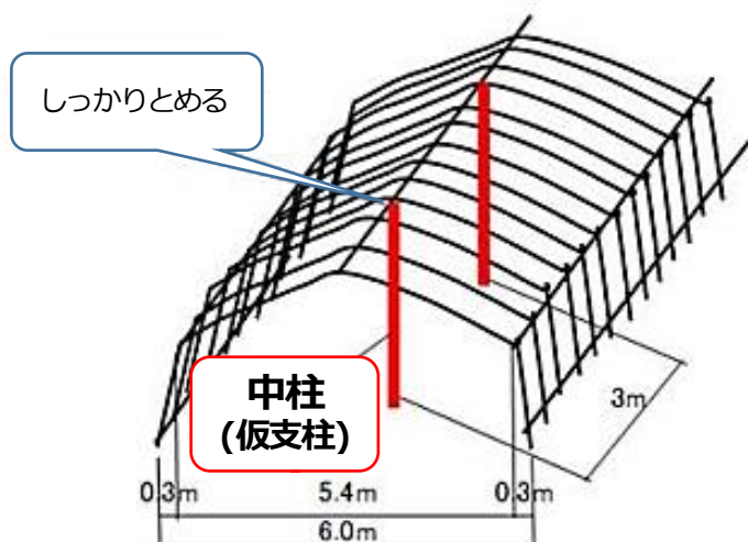
中柱（仮支柱）による補強事例
