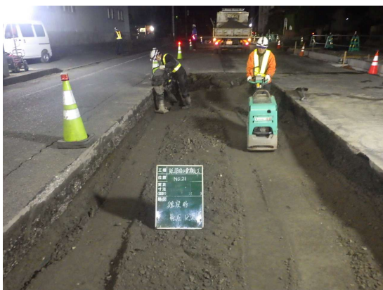
既設雨水管撤去 埋戻し状況
