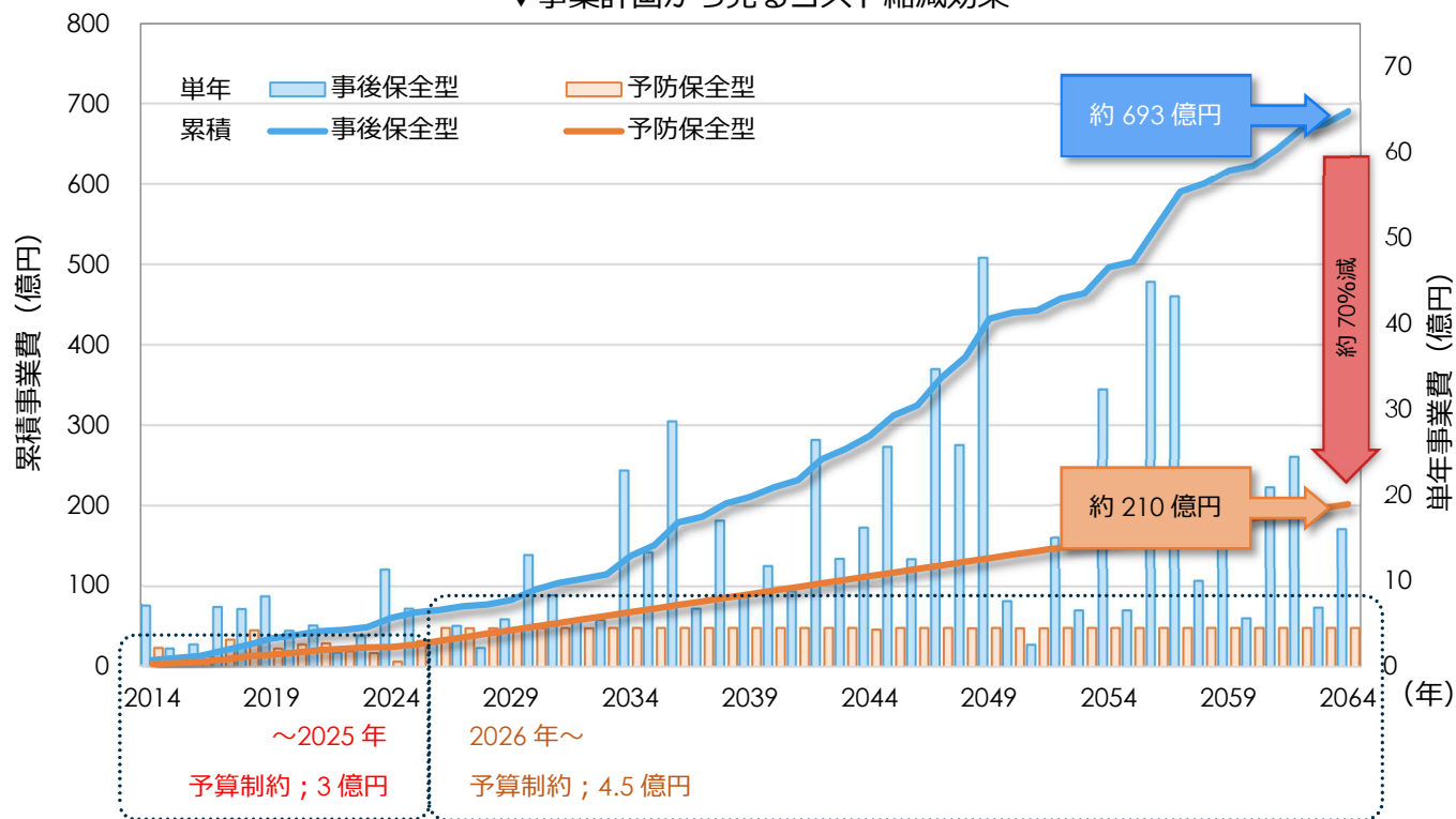
▼事業計画から見るコスト縮減効果
