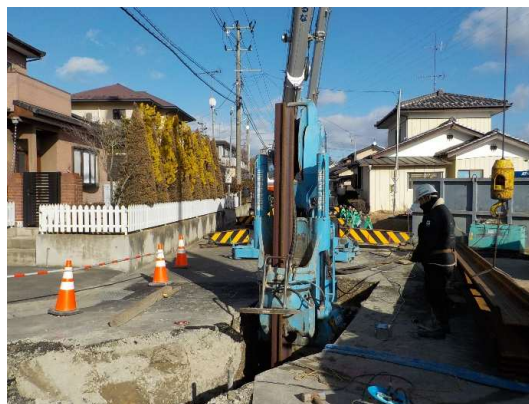
鋼矢板打ち込み状況
