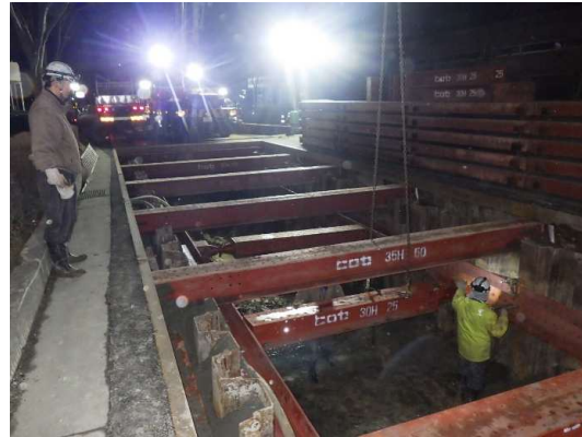
切梁設置状況
