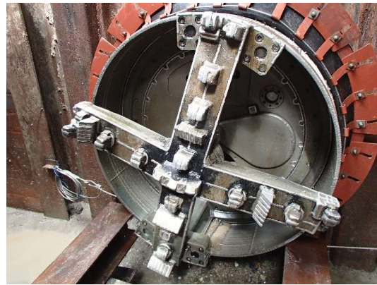
到達立坑内部 推進機到達状況
