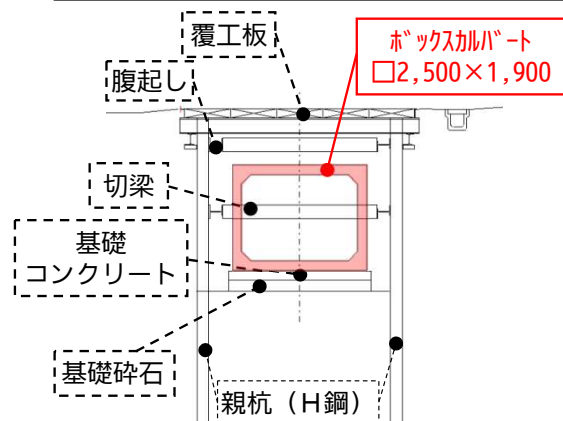
断面図
