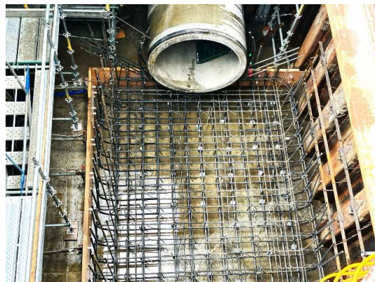
到達立坑：特殊人孔鉄筋組立状況
