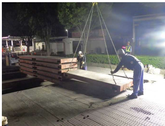
覆工板撤去状況
