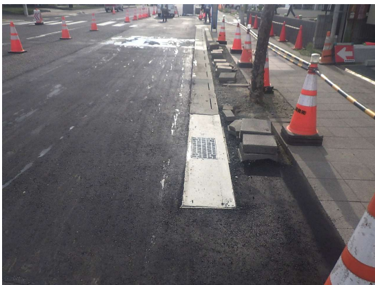
路面排水溝設置完了
