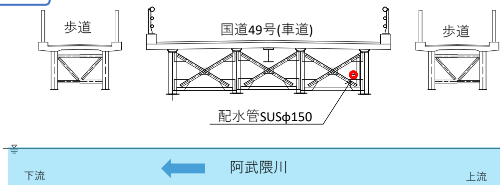
断面図
