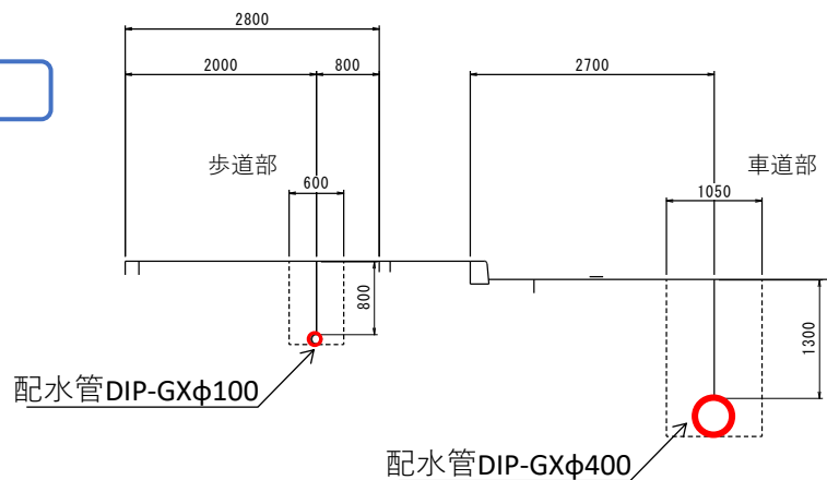
断面図
