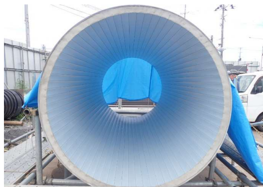
割込人孔・貯留管との接続管 (内面施工完了)
