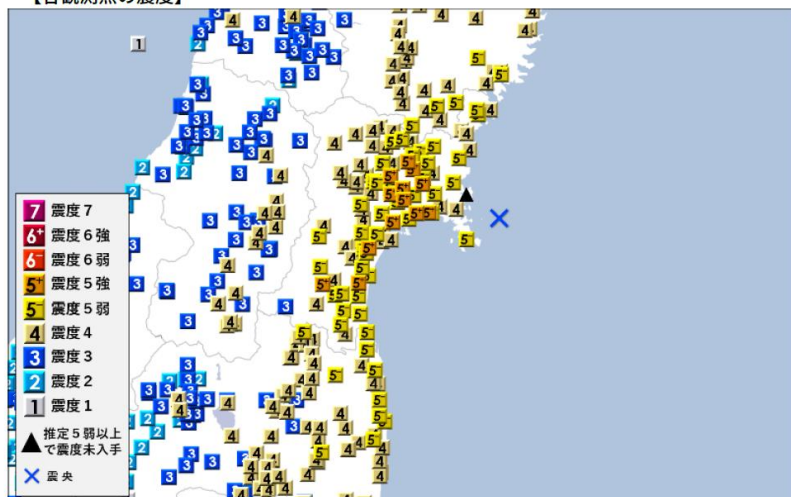
【各観測点の震度】
