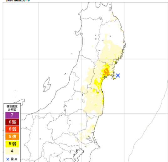
推計震度分布
