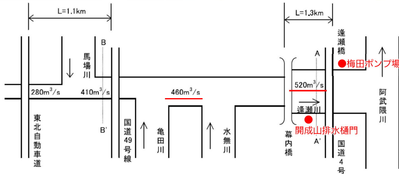
計画流量配分図(逢瀬川)
