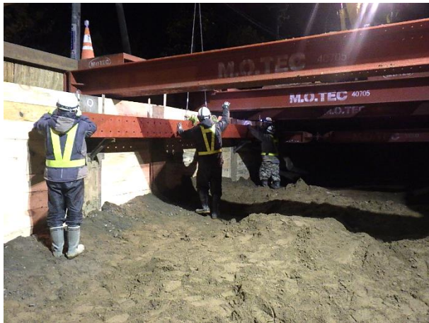
仮設土留(親杭(H鋼)横矢板工法)設置状況
