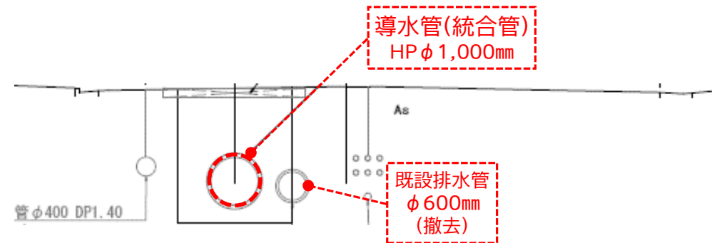
計画断面図
