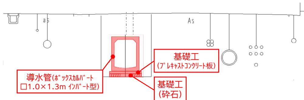
計画断面図
