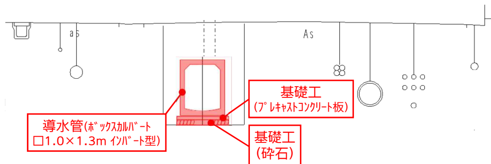
計画断面図
