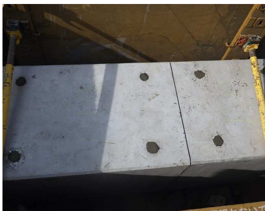
ボックスカルバート布設完了状況
