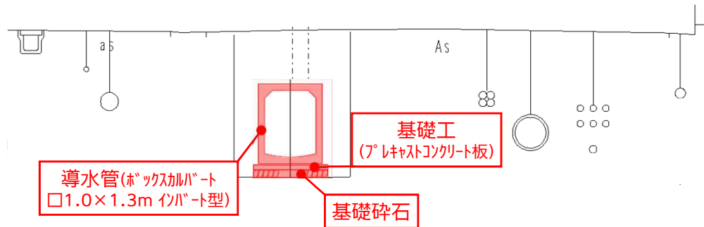
計画断面図
