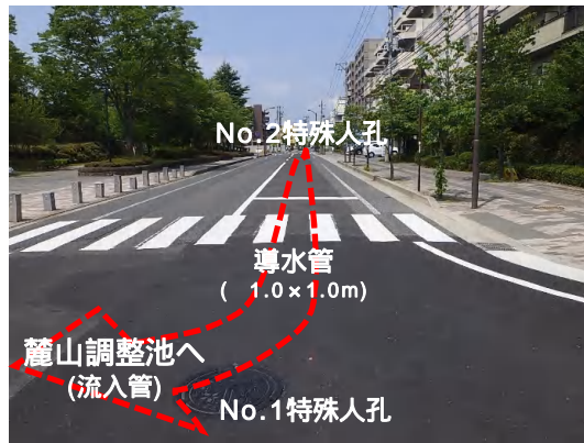
舗装仮復旧完了(No.1から上流を望む)
