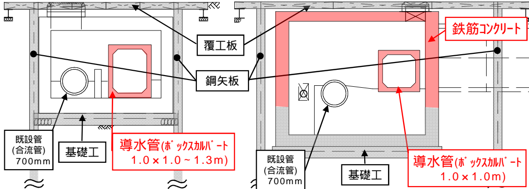
(No.2特殊人孔)計画断面図
