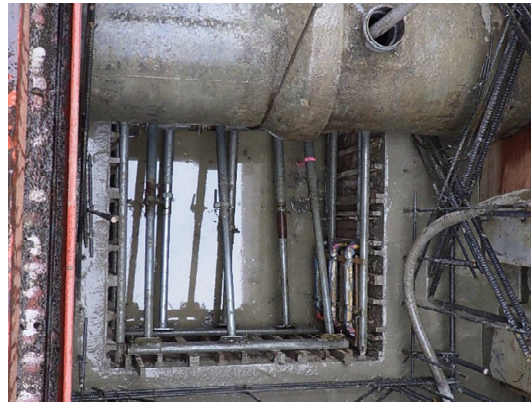
コンクリート打設状況(No.1特殊人孔)
