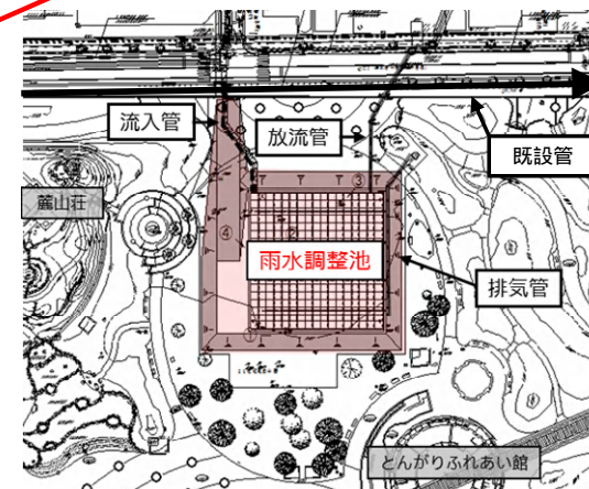
計画平面図(21世紀記念公園内)
