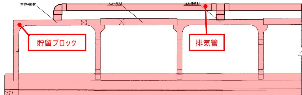
断面図(21世紀記念公園内)
