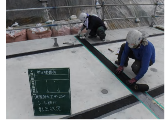
貯留ブロックの防水工状況
