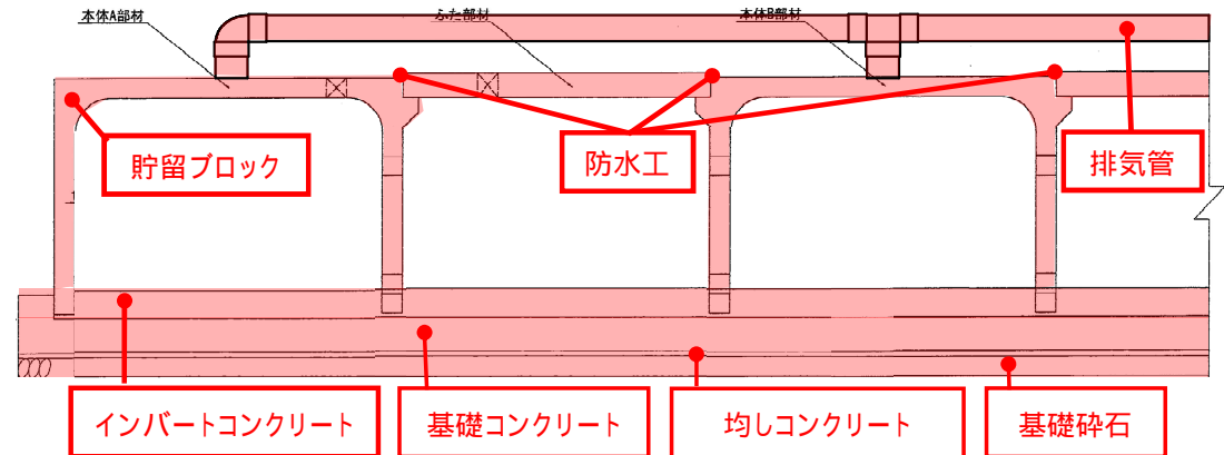
インバートコンクリート打設状況
