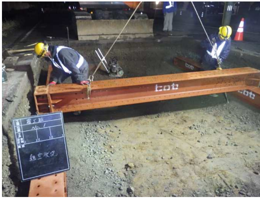
覆工板(受桁)設置状況
