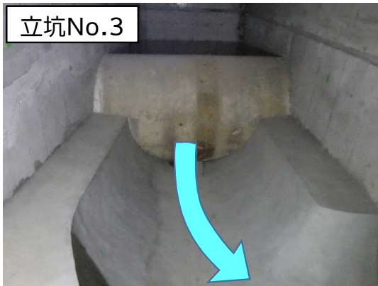
特殊人孔築造(ｲﾝﾊﾞｰﾄ)状況(上流側を望む)
