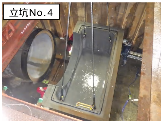
特殊人孔築造(基礎ブロック設置)状況
