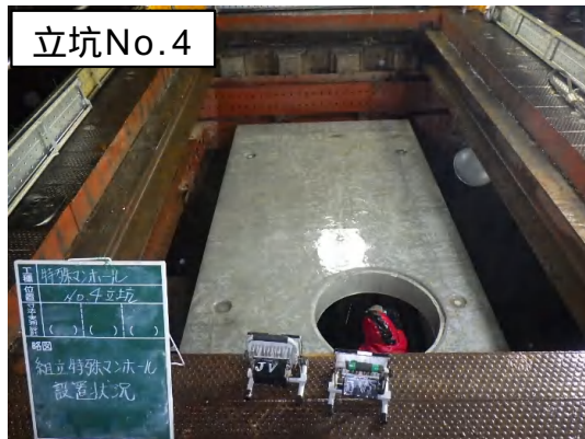
特殊人孔築造(頂版ブロック設置)状況
