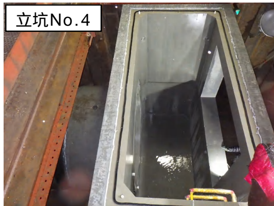
特殊人孔築造(中間ブロック設置)状況
