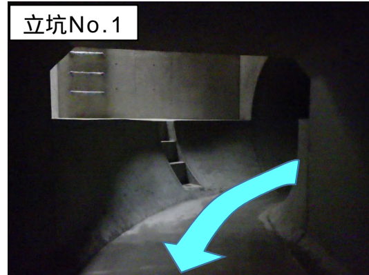
特殊人孔築造(バルト)状況(上流側を望む)
