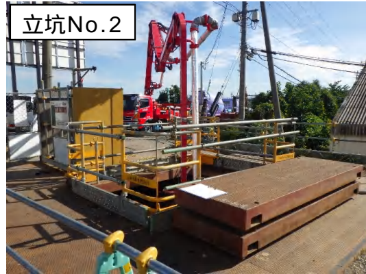
躯体コンクリート打設状況
