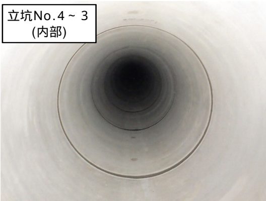
推進工法(ヒューム管布設完了)状況
