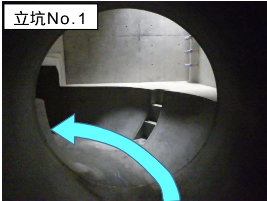
特殊人孔築造(バルト)状況(下流側を望む)
