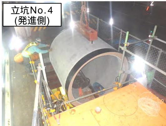
推進工法(ヒューム管投入)状況
