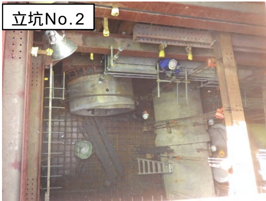
特殊人孔築造(底盤配筋)状況
