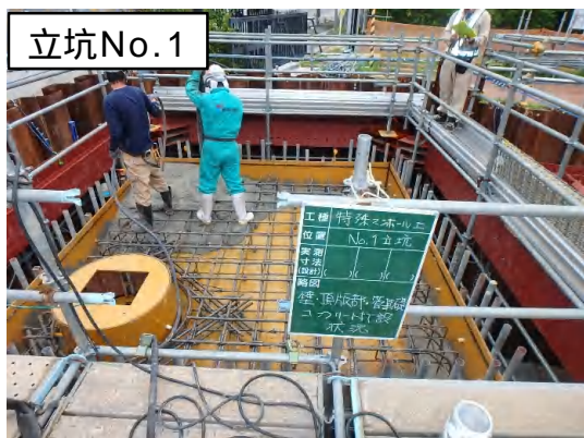
コンクリート打設(配筋)状況
