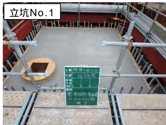
コンクリート打設状況
