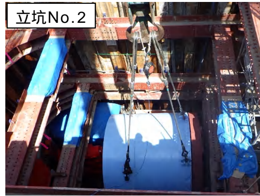
掘進機据付状況
