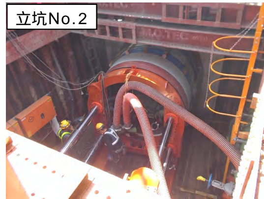
推進工法(U-M管布設)状況
