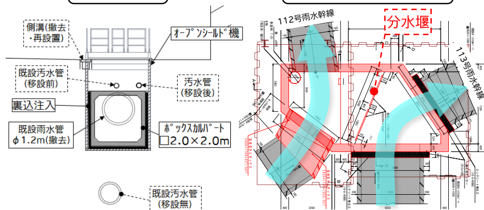
断面図
