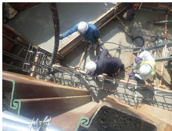
分水人孔(1次施工分)築造(コンクリート打設)状況
