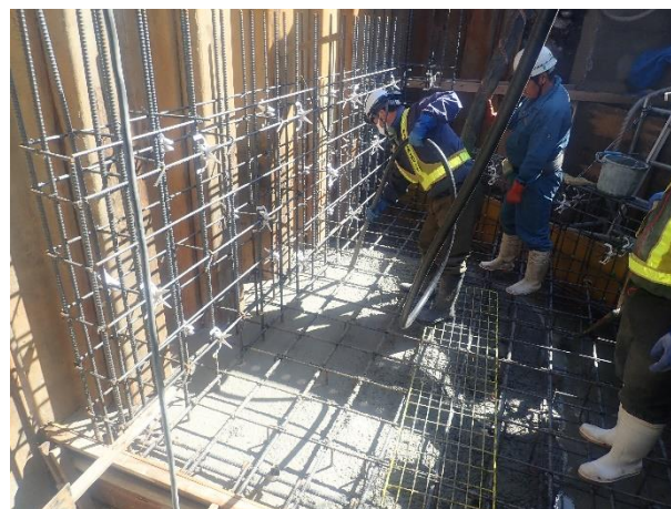
分水人孔築造(底版コンクリート打設)状況
