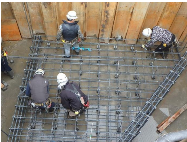
分水人孔築造(底版配筋)状況
