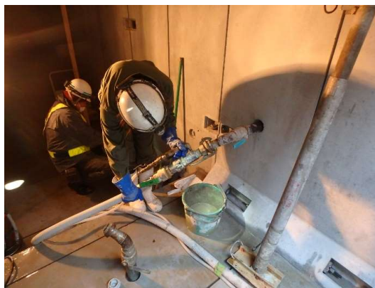
ボックスカバート布設(裏込注入)状況
